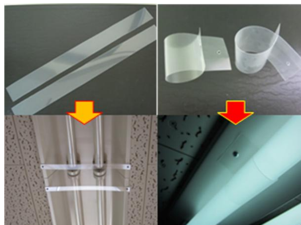
埋込型 と 露出型 蛍光管落下防止器具
